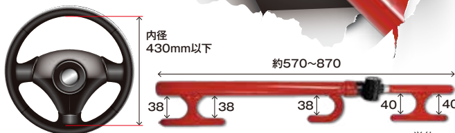
内径430mm以下のステアリングにご使用ください。
