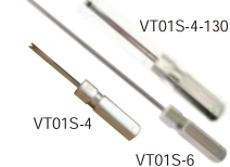
VT01S-4-130 VT01S-4 VT01S-6 VT01S-4-130/材質:スチール 全長:130mm 重さ:約34g VT01S-4/材質:スチール 全長:110mm 重さ:約33g VT01S-6/材質:スチール 全長:210mm 重さ:約50g
